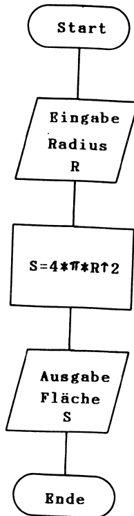
Programmablaufplan
